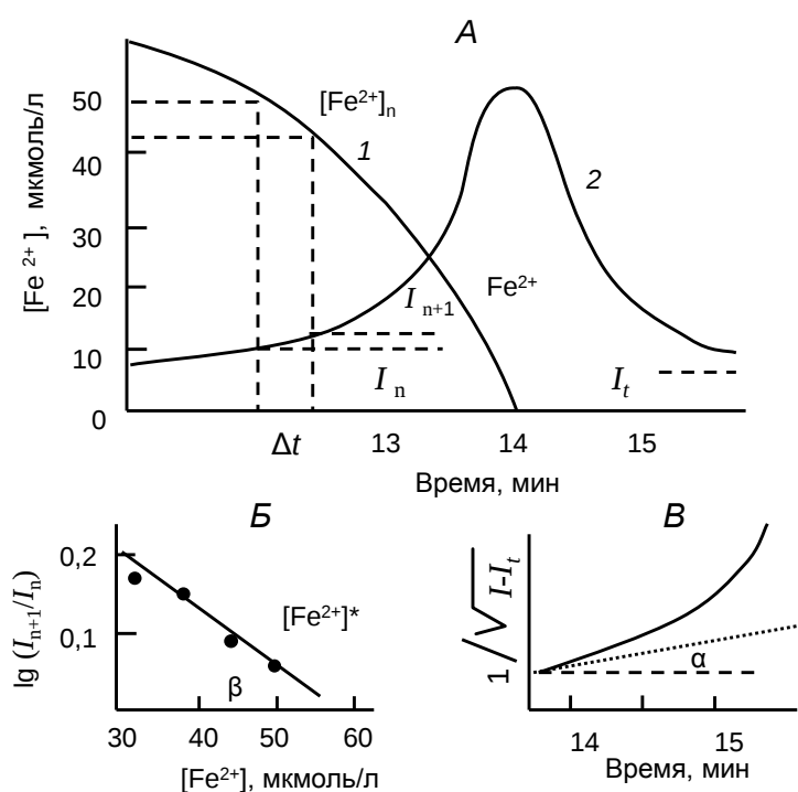
Рис. 5.18. Экспериментальное определение констант скоростей частных реакций, участвующих в процессе перекисного окисления липидов. А — кинетика изменения концентрации ионов железа [\text{Fe}^{2+}] (кривая 1) и хемилюминесценции I (кривая 2), В — нахождение константы скорости k_p и критической концентрации ионов железа [\text{Fe}^{2+}]^* . В — определение константы скорости k_6 (объяснения см. в тексте).
