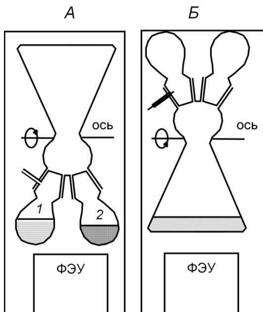
Рис. 5.15. Схема эксперимента для изучения быстрой вспышки хемилюминесценции.
