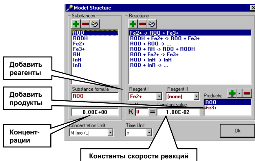
Рис. 5.20. Окно программы Kinetic Analyzer
