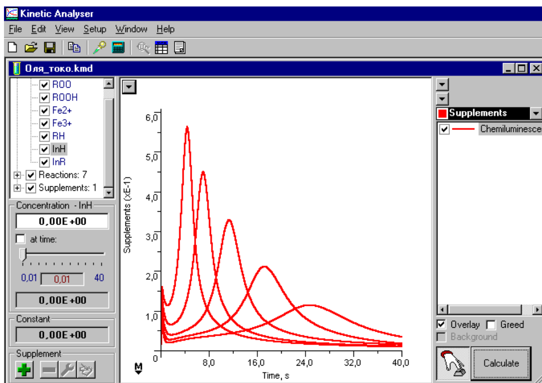
Рис. 5.21. Окно программы Kinetic Analyzer
