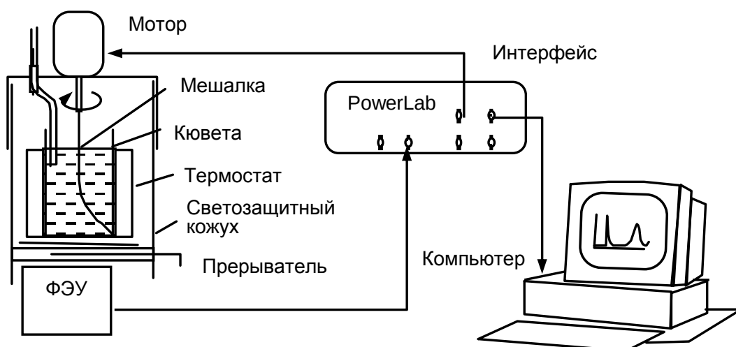
Рис. 5.13. Установка для измерения кинетики хемилюминесценции.
